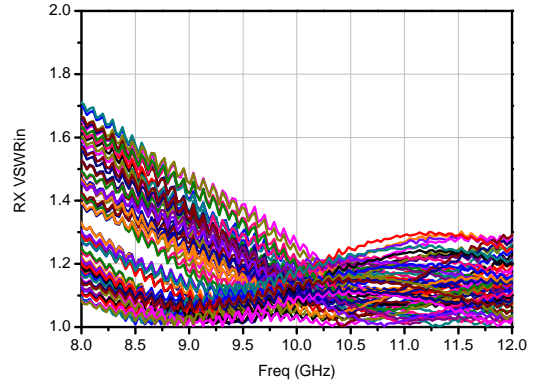
输入驻波
