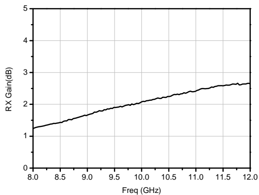
接收增益
