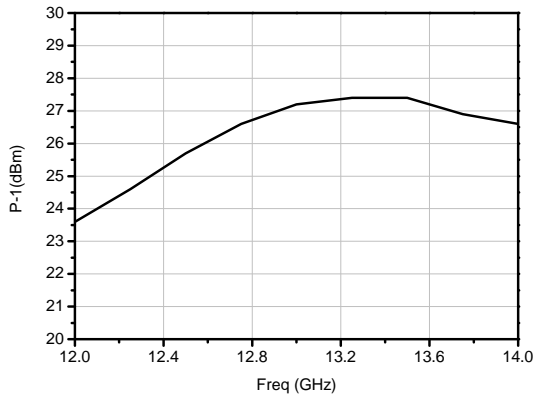
输出功率 (+6V)
