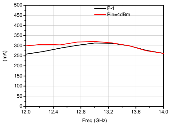
动态电流 (+6V)
