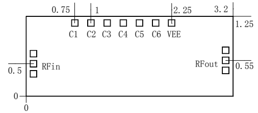
推荐装配图
