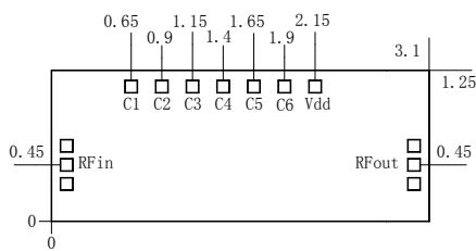
外形和端口尺寸 (mm)
