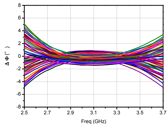
移相精度
