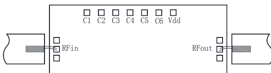
推荐装配图
