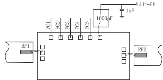
推荐装配图
