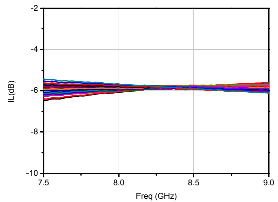
移相精度
