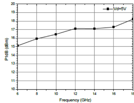
1dB 压缩点输出功率
