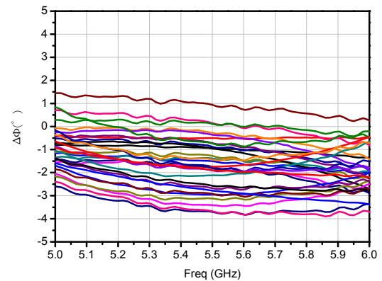
移相精度
