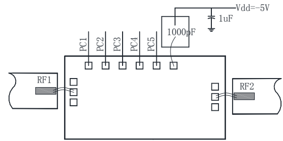
推荐装配图
