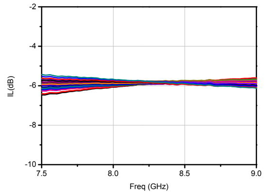
移相精度
