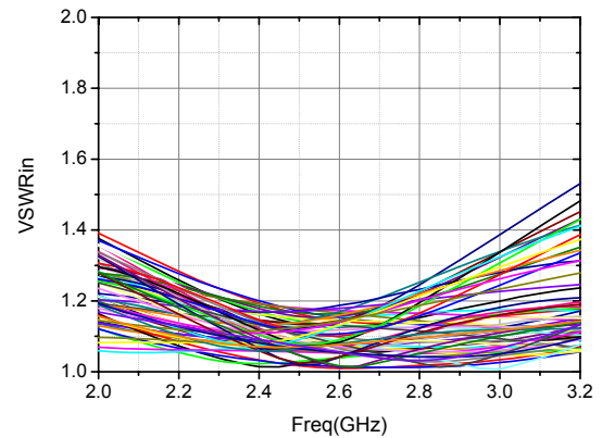
Input VSWR
